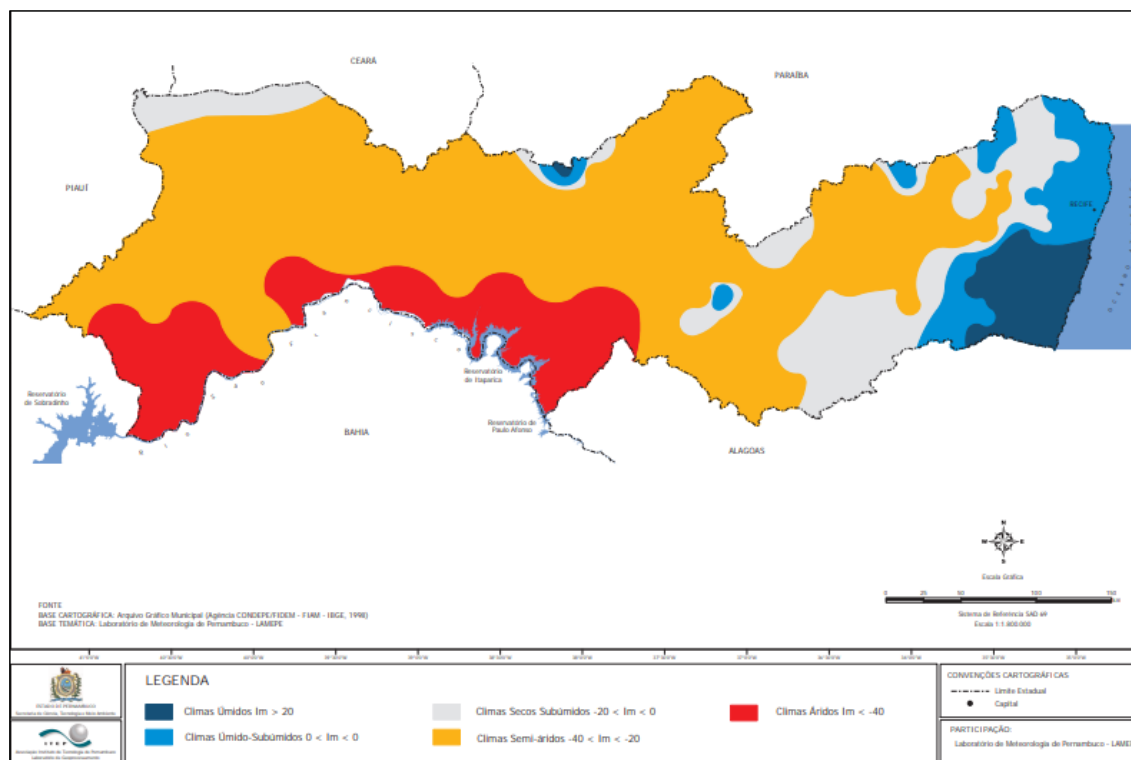
Figura: Clima de Pernambuco
