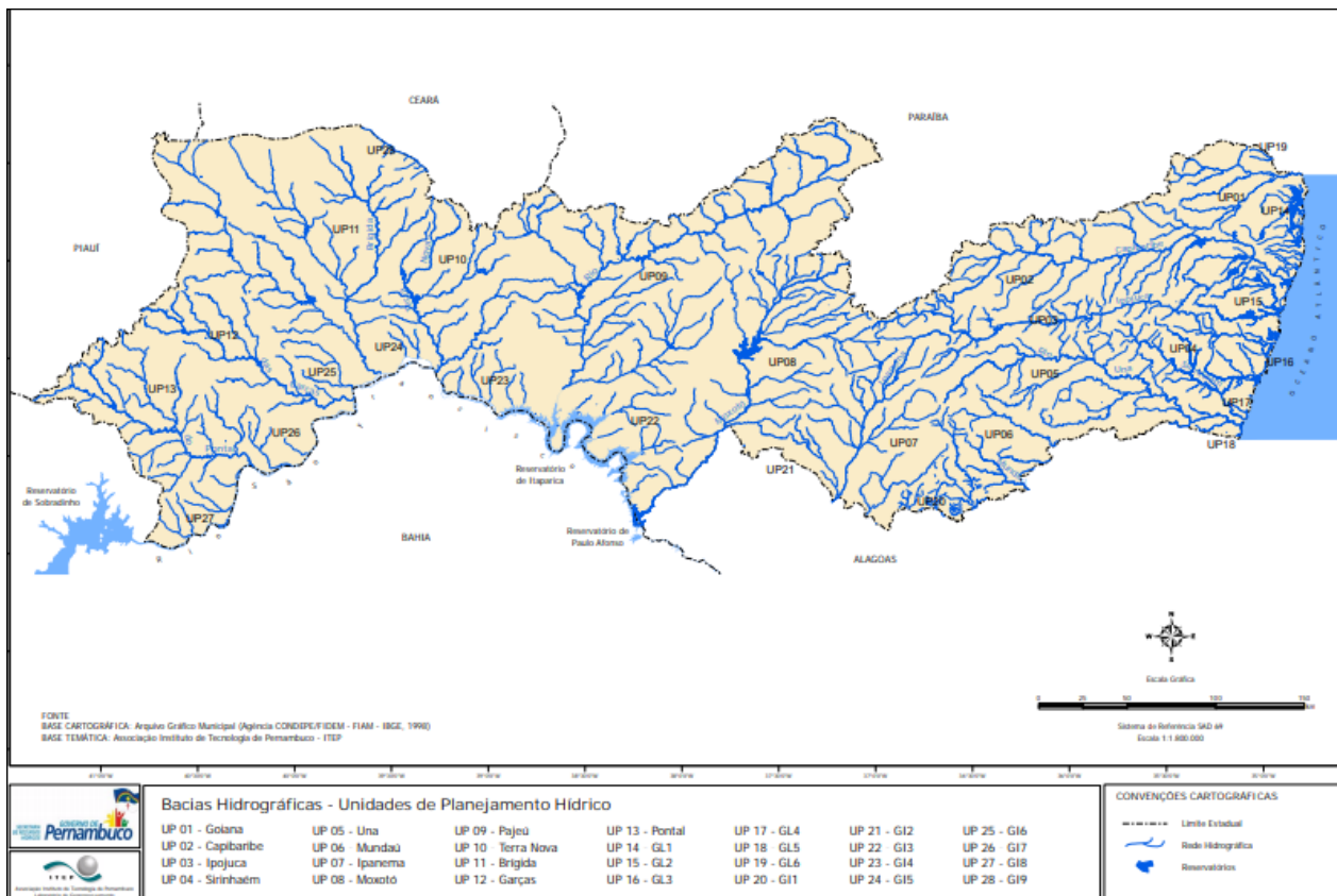
Figura: Hidrografia de Pernambuco
